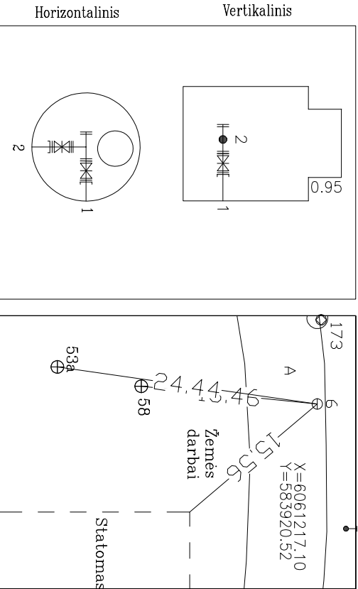
ŠULINIO PĖLYVAI (Matavims duoti m)
