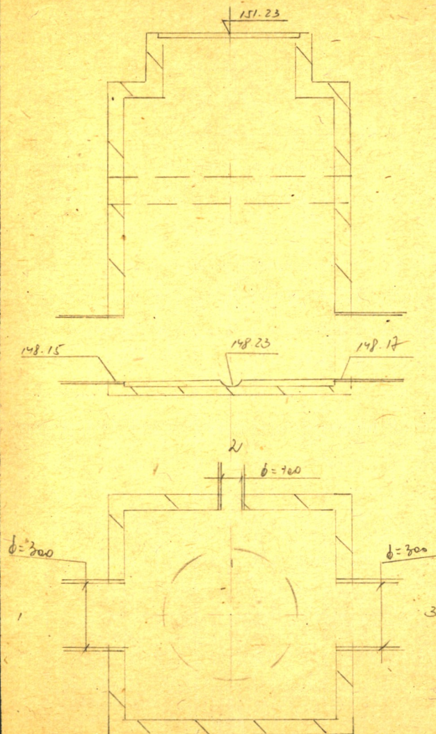
Чертеж колодца М 1:
