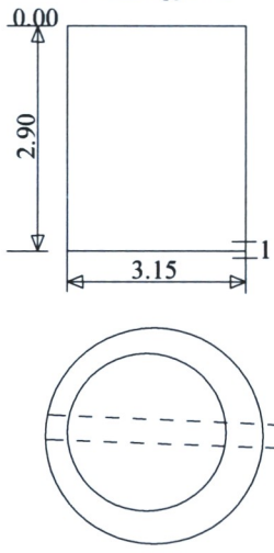
Šulinio pjūvis
