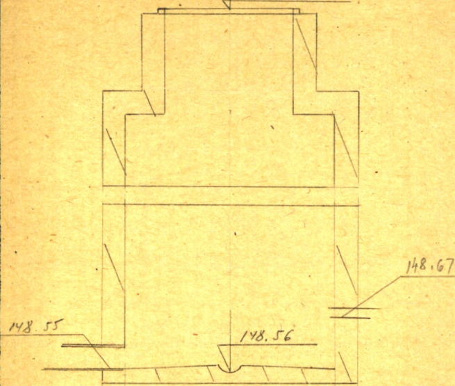
Чертеж колодца М 1: 150.98
