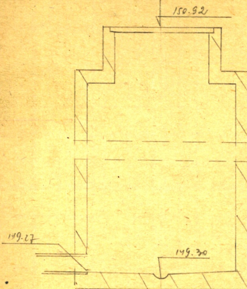
Чертеж колодца М 1:
