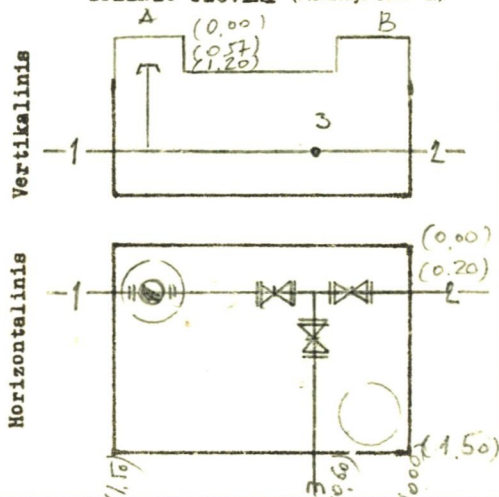
ŠULINIO PIŪVIAI (Matmenys duotai m)
