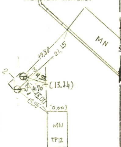
PRIRIŠIMO BRĖŽINYS
