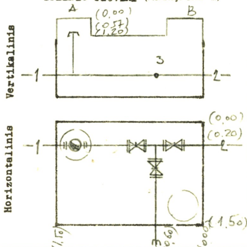
ŠULINIO PIŪVIAI (Matmenys duoti m)
