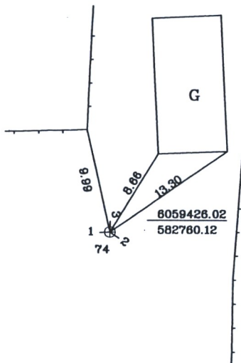
Pririšimo brėžinys
