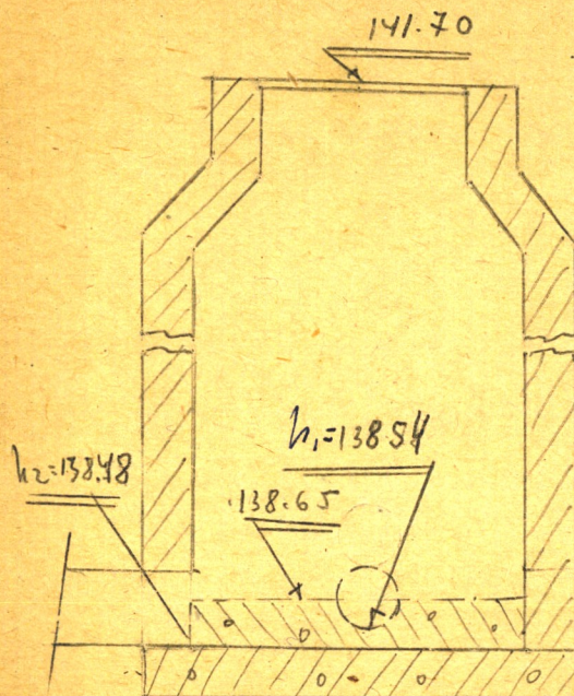
Чертеж колодца М 1:
