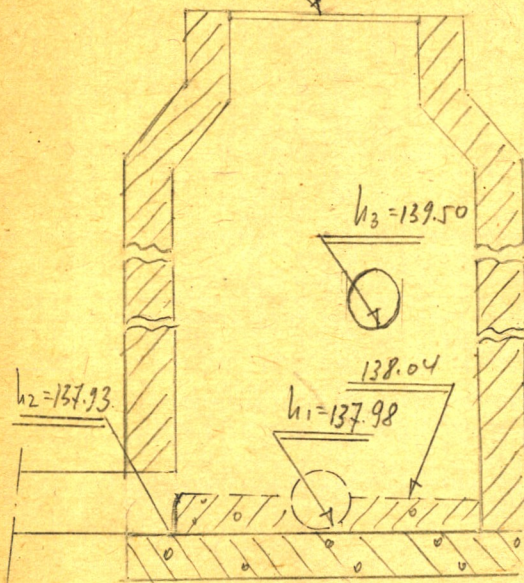
Чертеж колодца М 1:25 141.32
