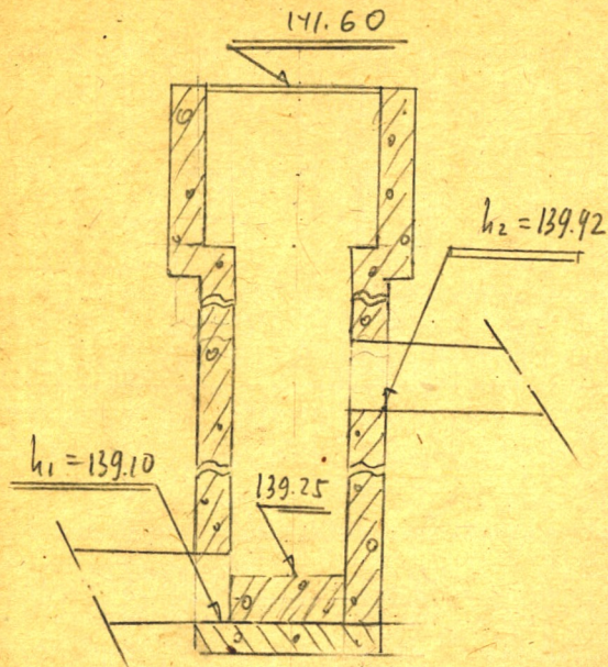
Чертеж колодца М 1:25
