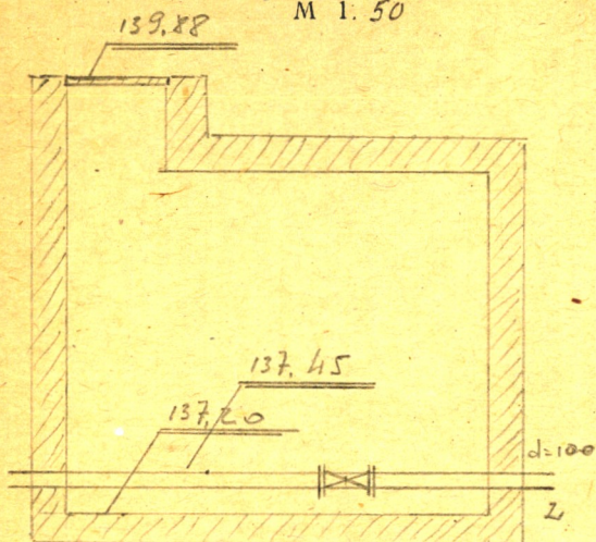
Чертеж колодца М 1:50
