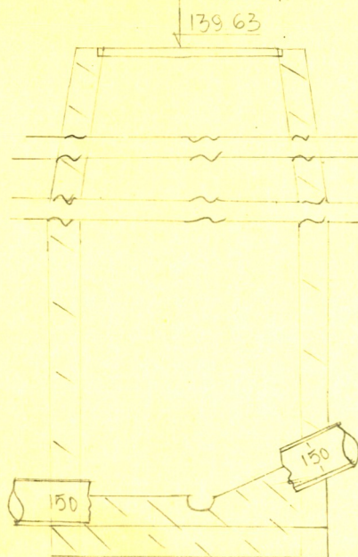
Чертеж колодца М 1:25 от А-А
