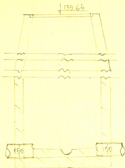
Чертеж колодца М 1:25 по А-А
