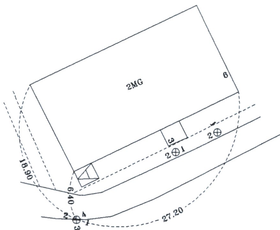
Pririšimo brėžinys
