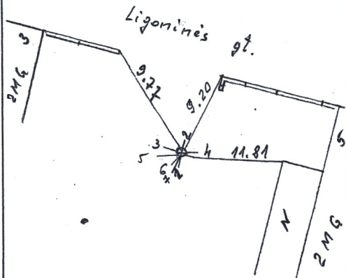
PRIRIŠIMO SCHEMA
