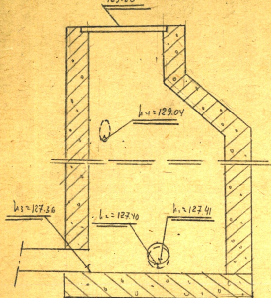
Чертеж колодца 129.80 М 1:25
