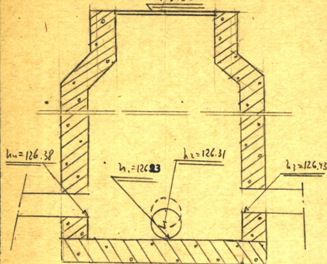
Чертеж колодца М 1:25 129.86
