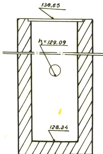
Чертеж колодца М1:25
