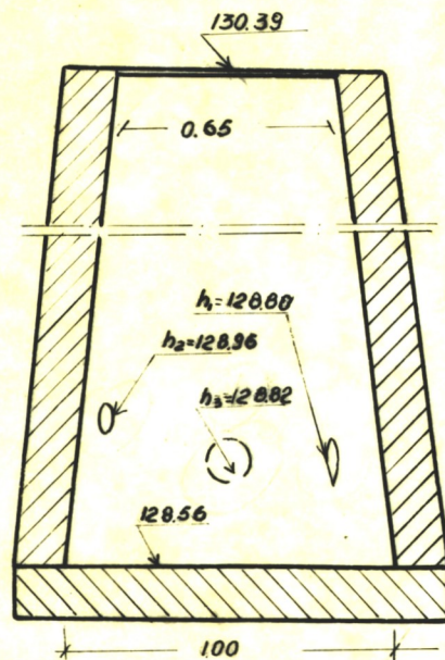
Чертеж колодца М 1:25
