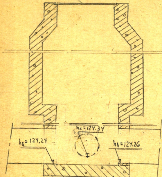
Чертеж колодца
