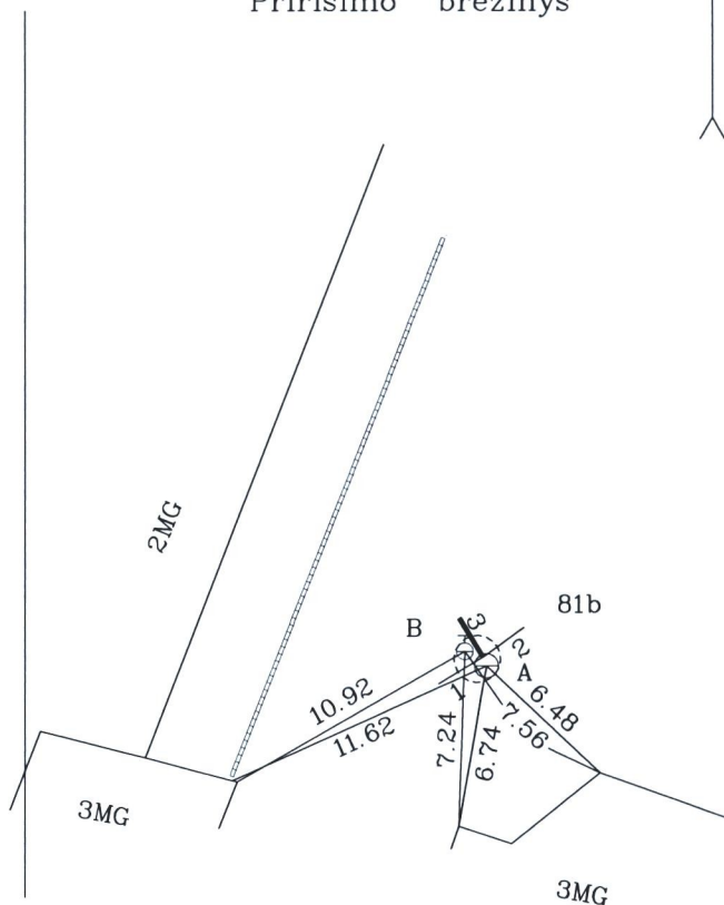
Pririšimo brėžinys
