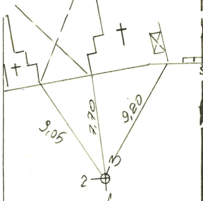
PRIRIŠIMO BRĖŽINYS
