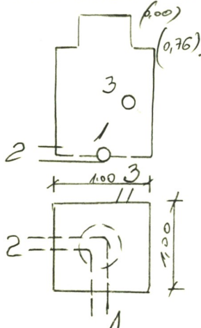
ŠULINIO PIŪVIAI (Matmenys duoti m)
