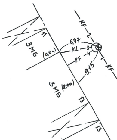
PRIRIŠIMO SCHEMA
