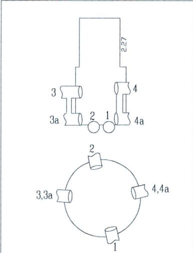
ŠULINIO PJŪVIAI (Matmenys duoti m)
