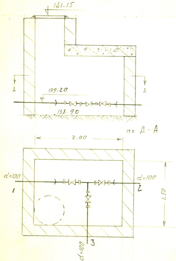
Чертеж колодца М. 1:50
