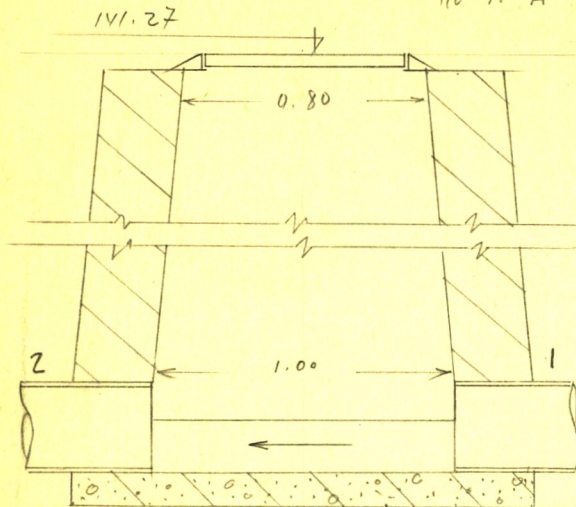
Чертеж колодца М 1:25
