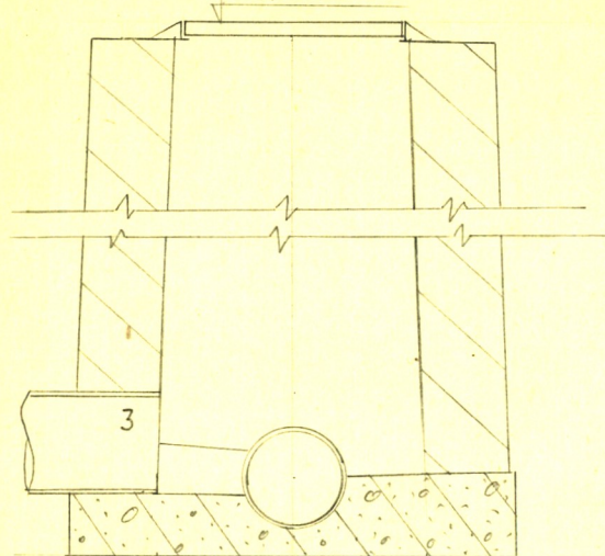
Чертеж колодца М 1:25 по А-А
