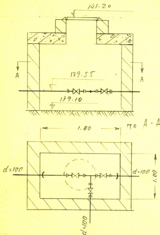
Чертеж колодца М. 1:50
