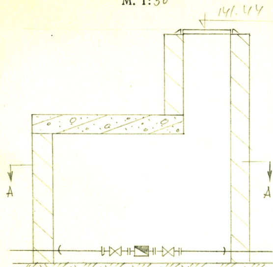
Чертеж колодца М. 1:50
