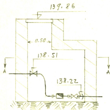
Чертеж колодца М. 1:50
