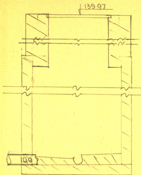
Чертеж колодца М 1:25 по А-А
