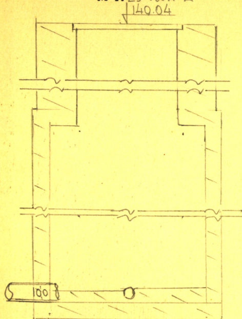
Чертеж колодца М 1:25 по А-А
