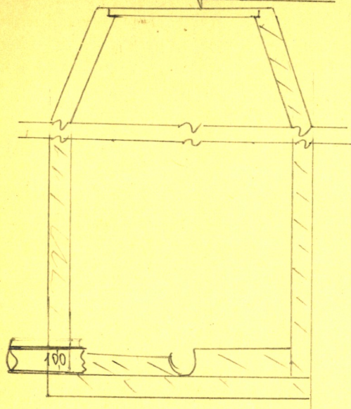
Чертеж колодца М 1:25 на А-А 140.03
