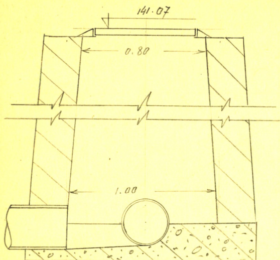
Чертеж колодца М 1:25
