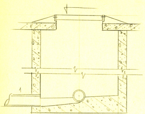
Чертеж колодца М 1: 25 Разрез по А-А
