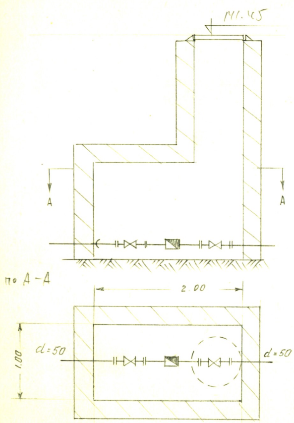
Чертеж колодца М. 1:50
