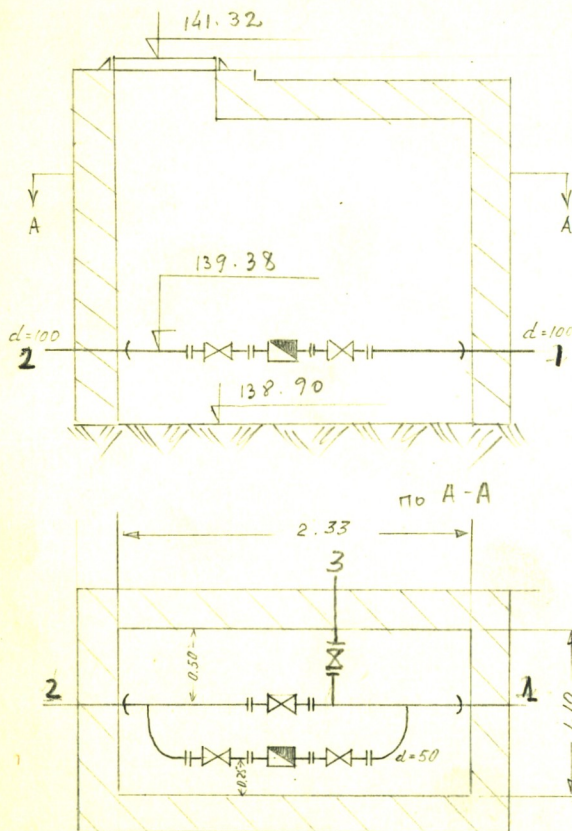
Чертеж колодца М. 1:50
