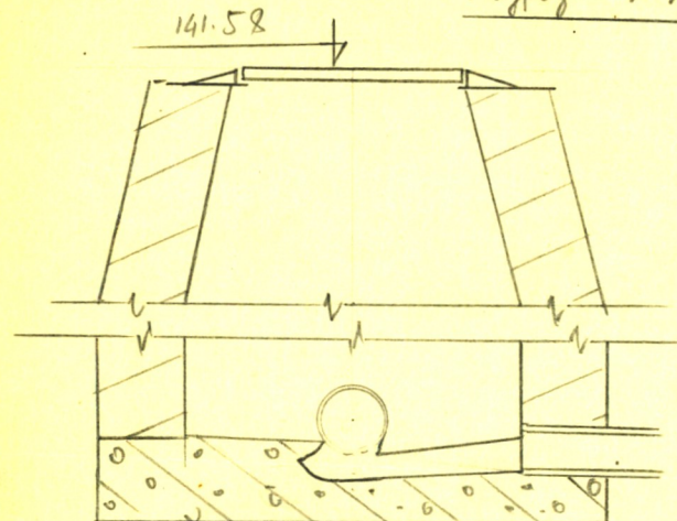
Чертеж колодца М 1:25
