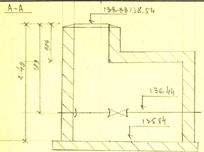
Чертеж колодца М 1:50
