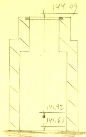
Чертеж колодца М. 1:50
