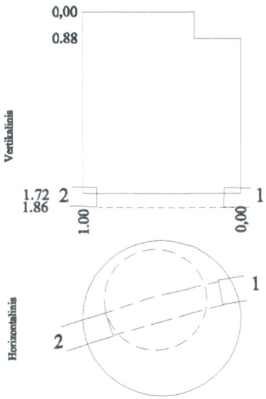
Šulinio pjūviai:
