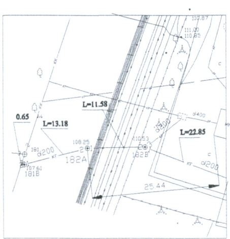
Pririšimo brėžinys:
