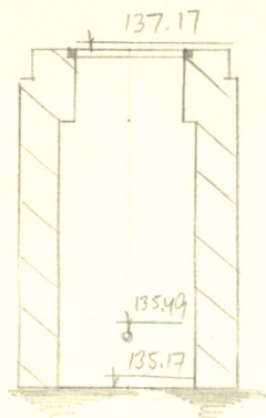
Чертеж колодца М. 1:50
