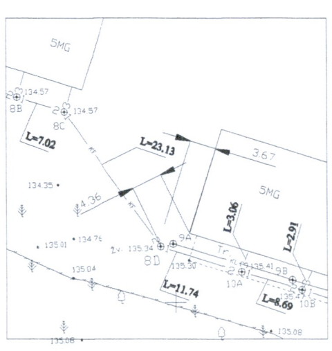
Pririškimo brėžinys:
