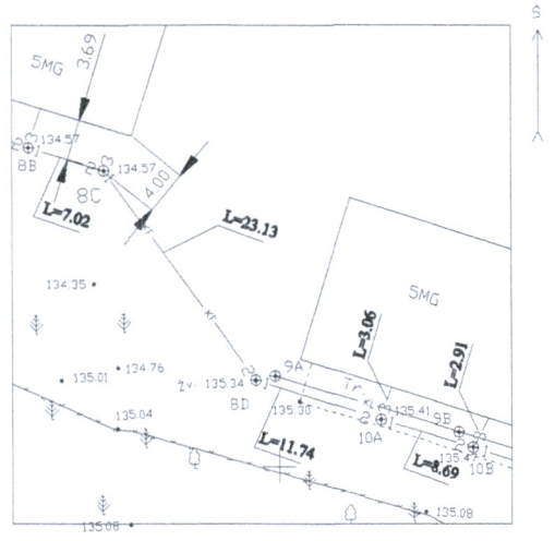
Pririšimo brėžinys:
