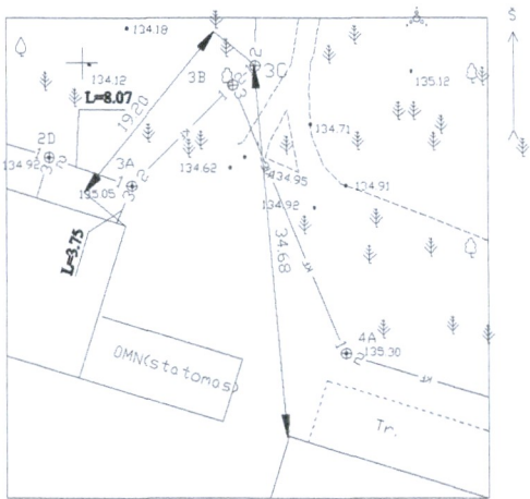
Pririšimo brėžinys:
