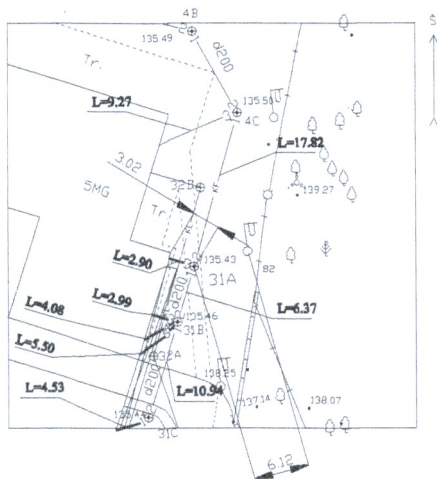
Prikirimo brėžinys:
