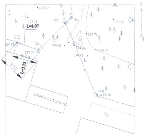
Pririšimo brėžinys:
