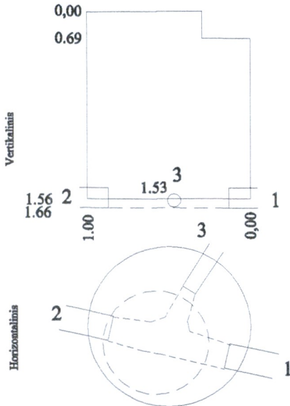
Šulinio pjūčiai:
