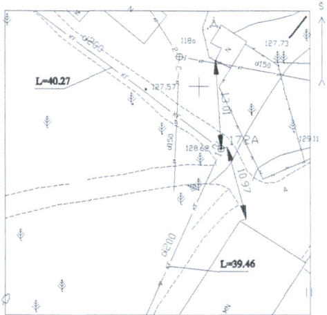
Pririšimo brėžinys:
