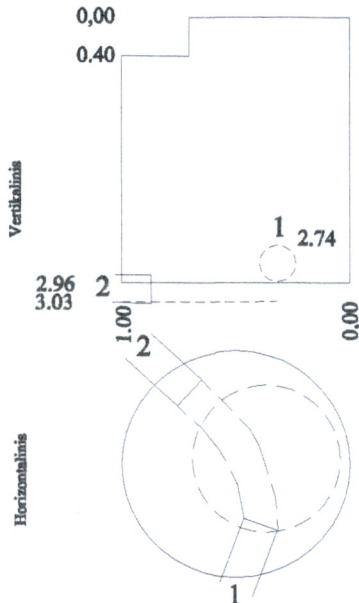
Šulinio pjūviai:
